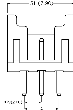
2x3Circuits
