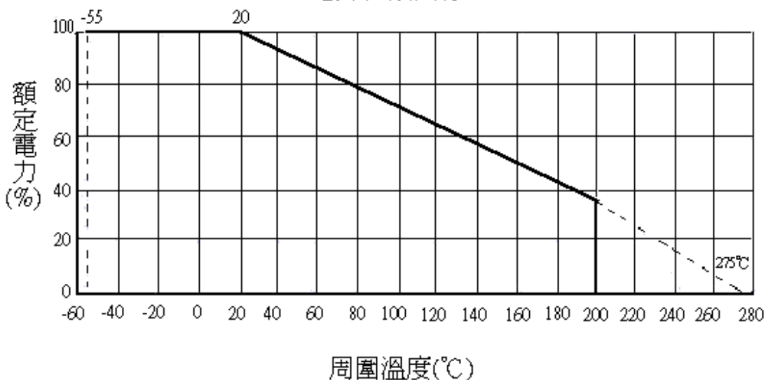
電力輕減曲線
