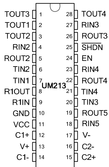
SOP28/SSOP28/TSSOP28
