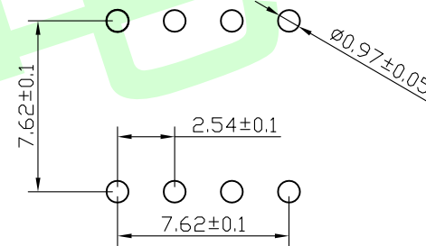
PCB开孔
