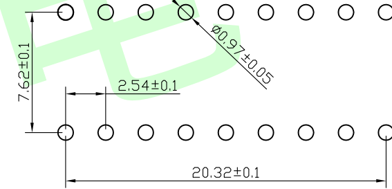
PCB开孔
