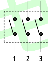
电路图
