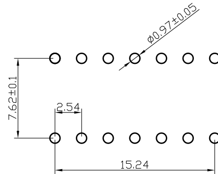
PCB开孔
