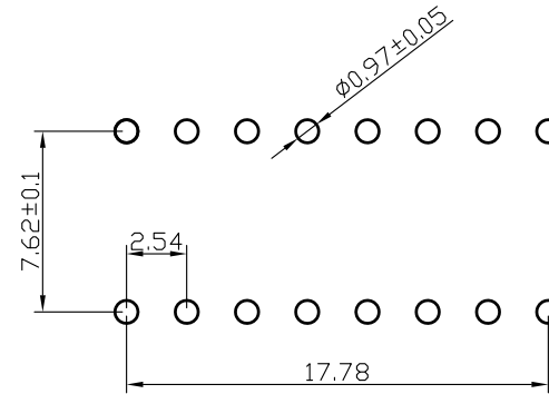
PCB开孔
