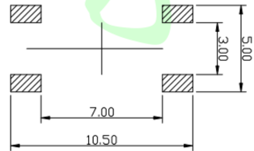
PCB. 焊接图
