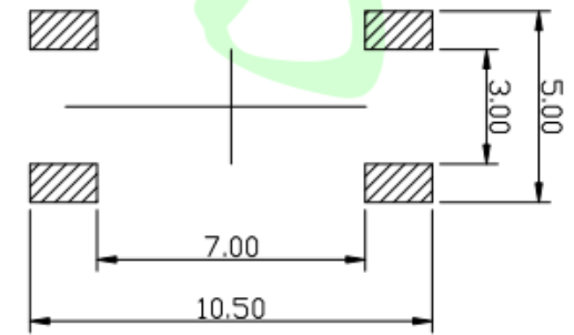
PCB. 焊接图
