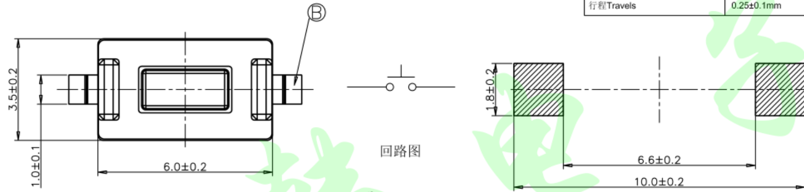
安装尺寸图
