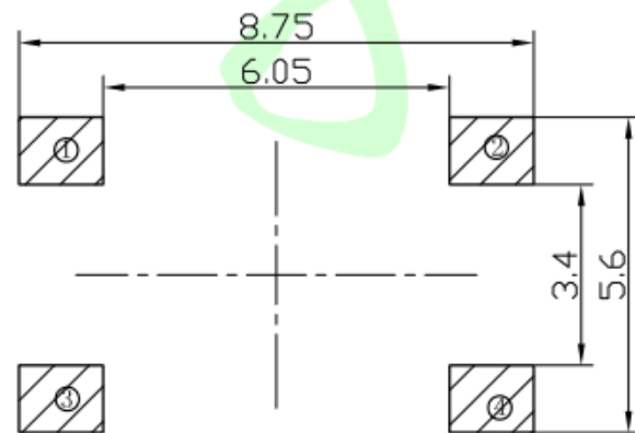
安装参考图
