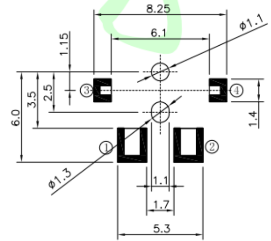
安装尺寸图
