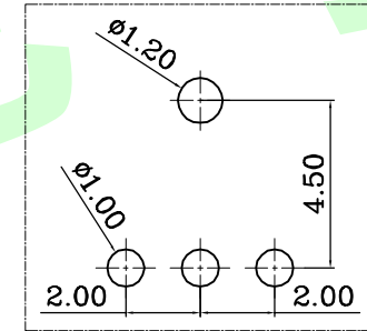
印刷电路板焊接处尺寸图
