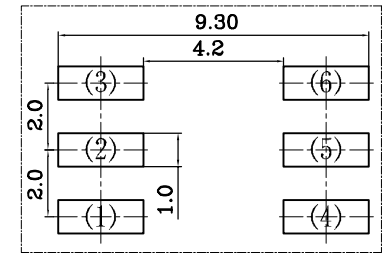
印刷电路板焊接处尺寸图
