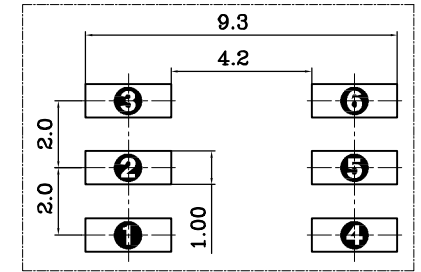
印刷电路板焊接处尺寸图
