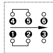
电路图
