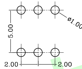
印刷电路板焊接处尺寸图
