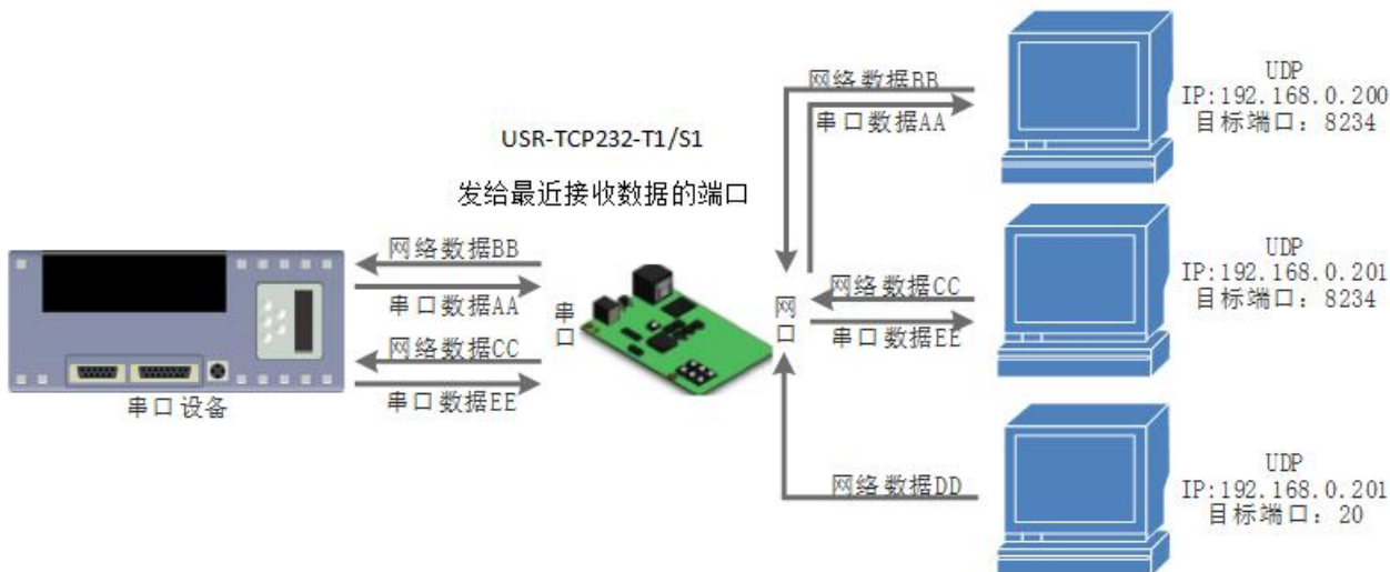
图 15. UDP Server 模式
