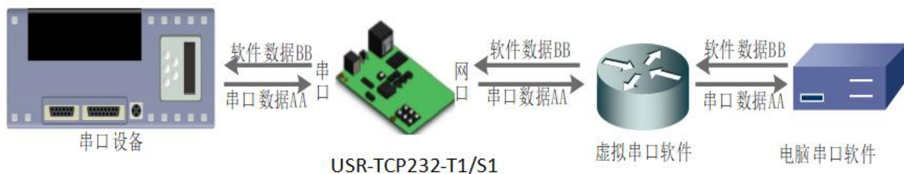
图 18. VCOM 应用示意图
