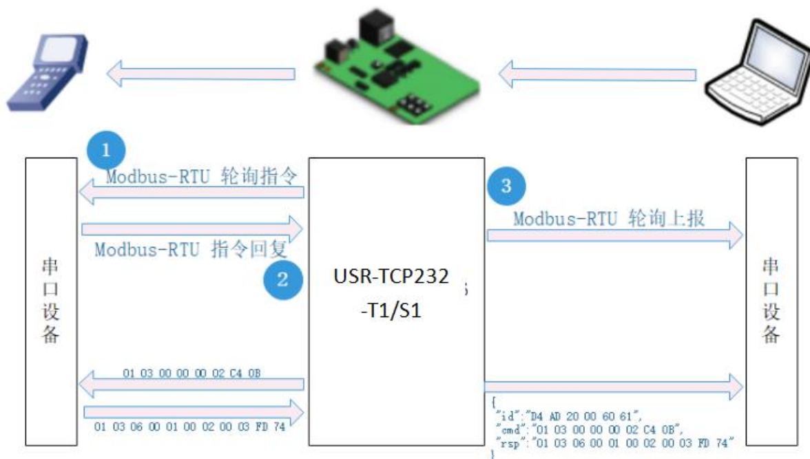
图 22. Modbus 采集轮询功能框图
