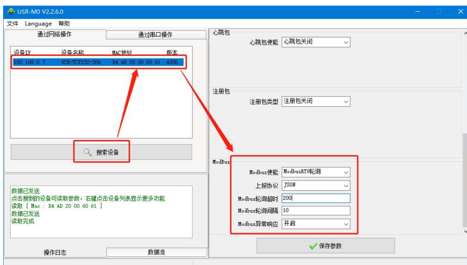
图 24. 软件设置 Modbus 协议轮询采集功能
