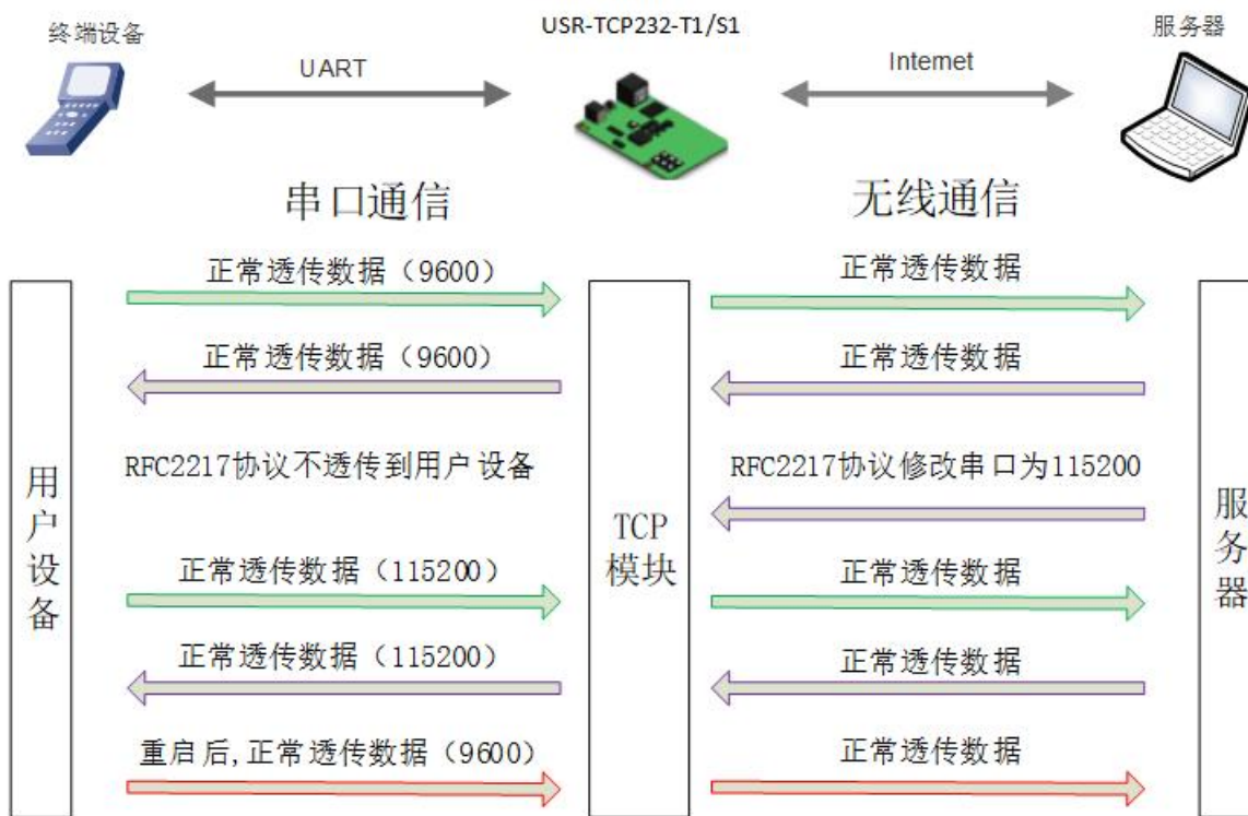
图 36. RFC2217 功能框图
