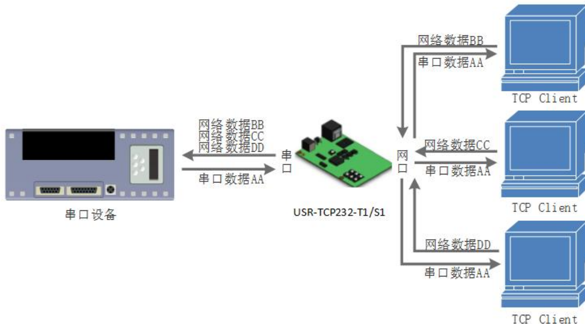
图 12. 图 15 TCP Server 模式说明
