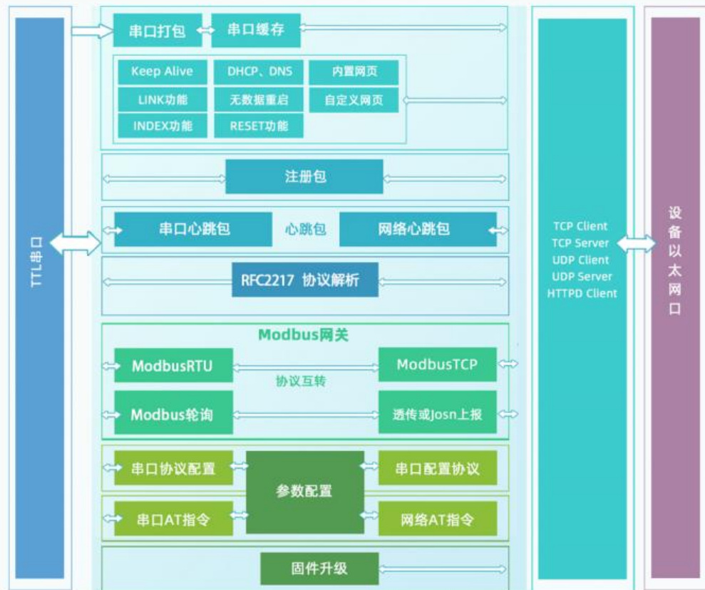
图 3. USR-TCP232-T1/S1 功能框图
