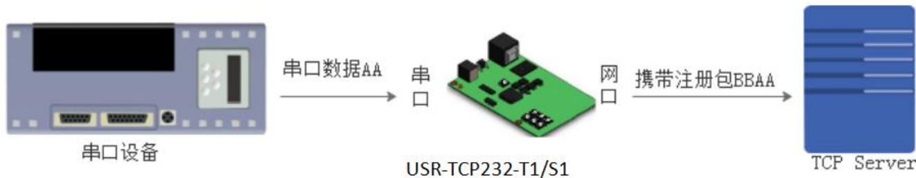
图 30. 数据携带注册包
