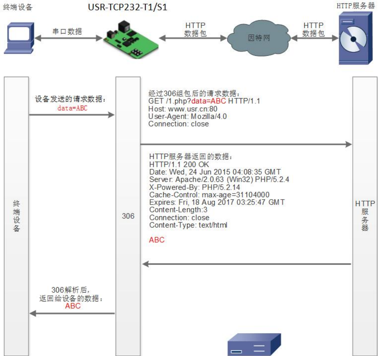
图 16. HTTPD Client 模式说明
