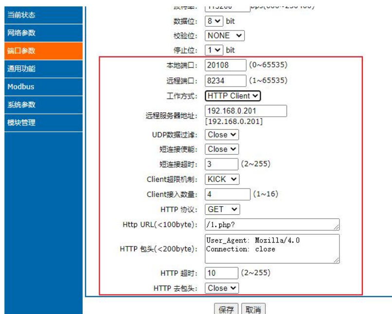
图 17. Httpd Client 设置图示
