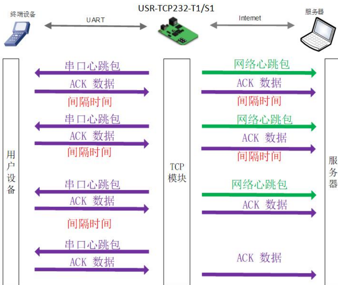
图 28. 心跳包功能示意图
