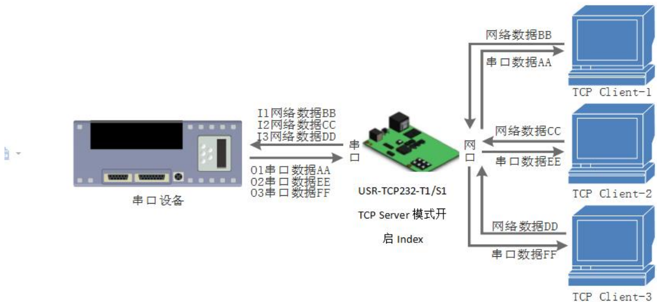
图 33. Index 功能示例图
