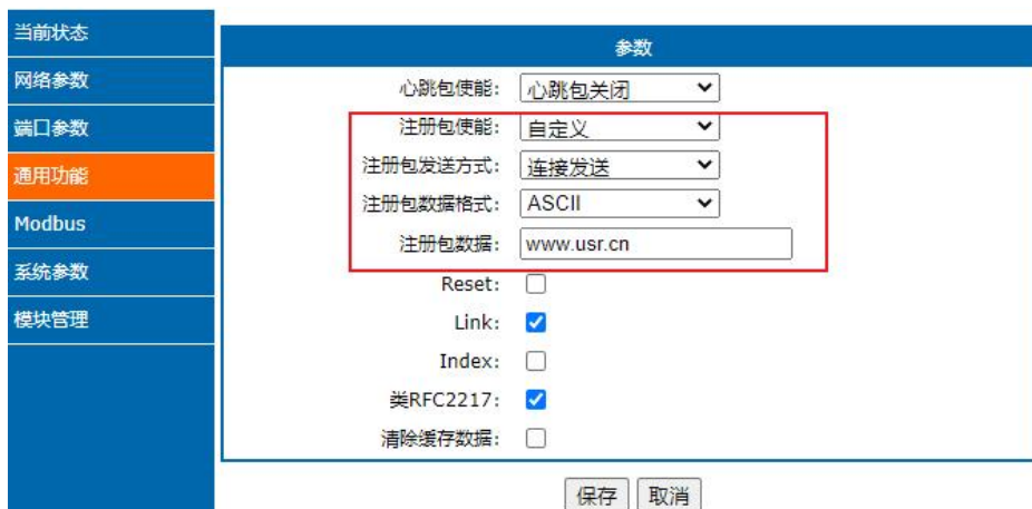
图 31. 注册包设置
