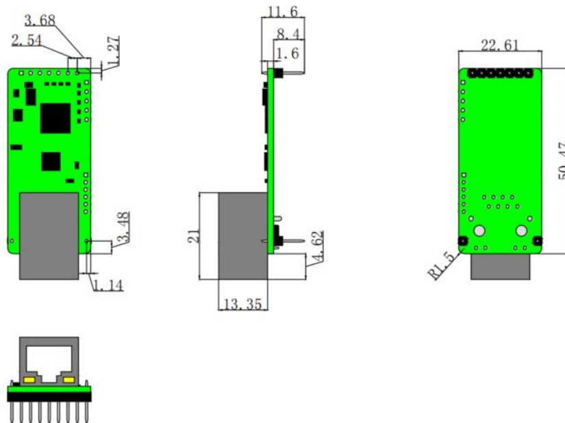
图 1. USR-TCP232-T1 尺寸图
