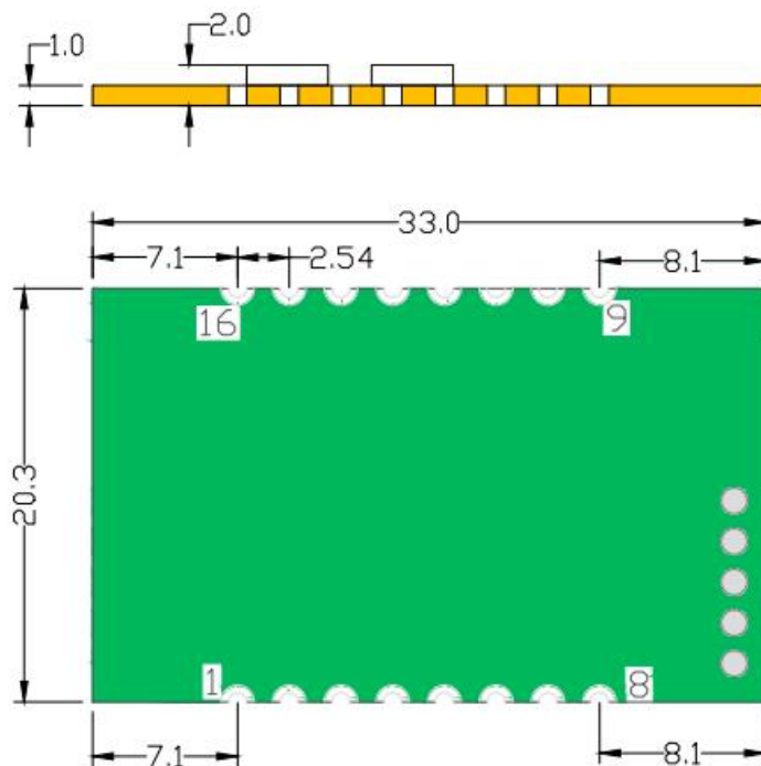
图 2. USR-TCP232-S1 尺寸图
