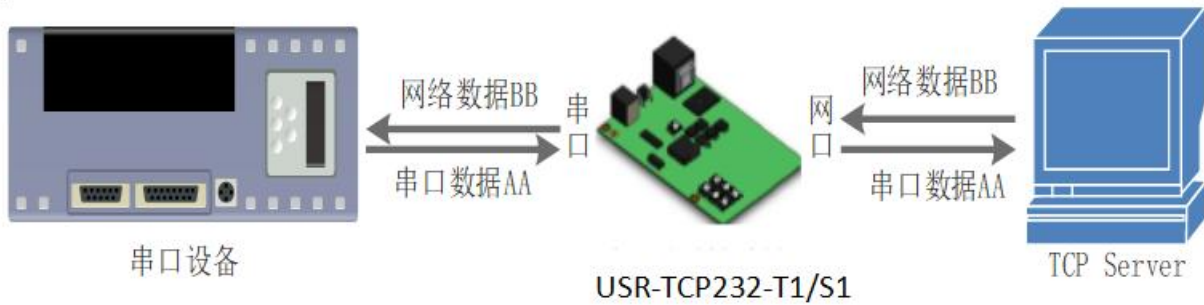
图 10. TCP Client 模式说明
