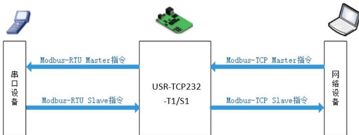
图 19. Modbus 协议转换功能框图
