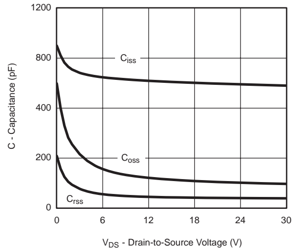
C_{iss}
