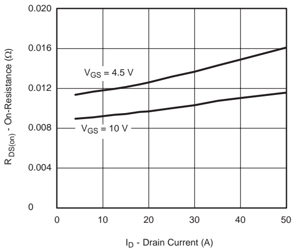
V_{GS} = 4.5 V
