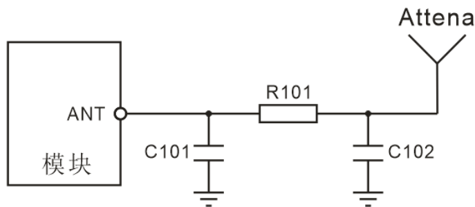
图 7-1 天线接口参考电路
