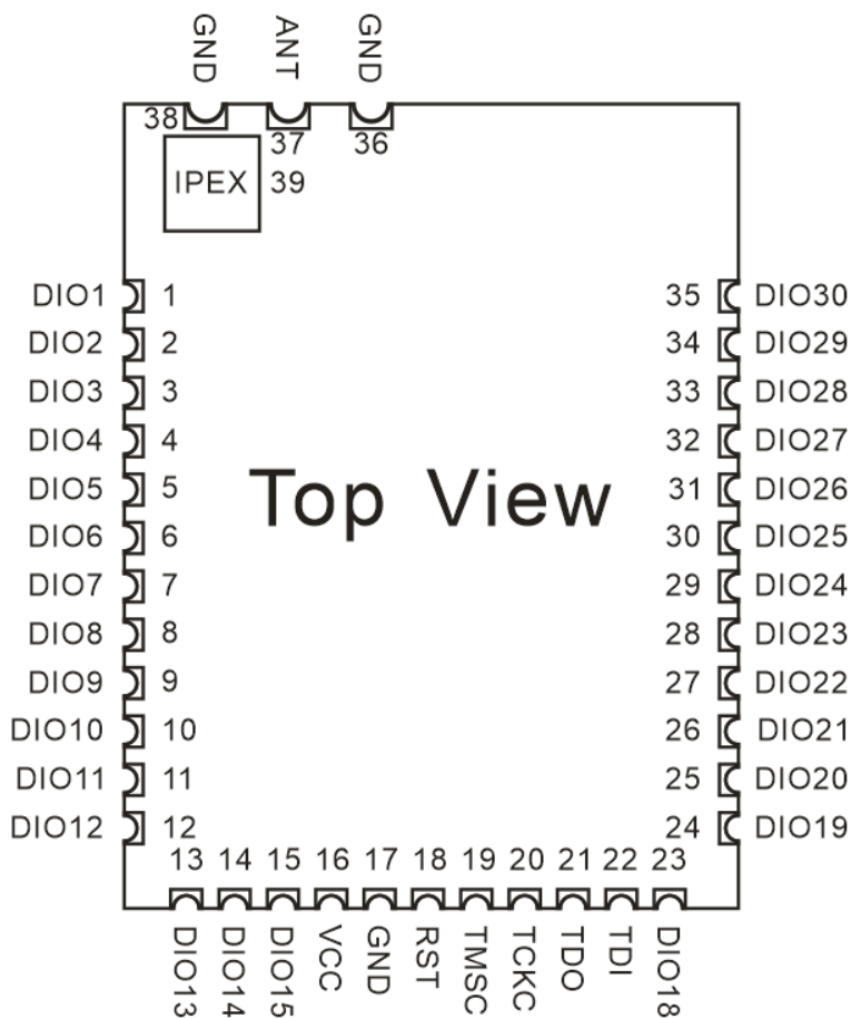
VT-S02A 尺寸 21.0 × 16.0 mm，引脚间距 1.27mm
