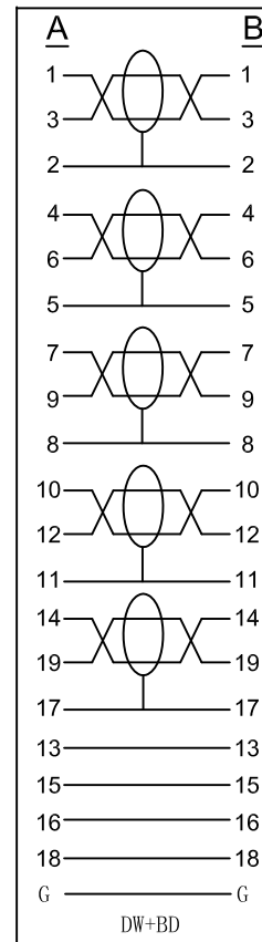
WIRING DIAGRAM:
