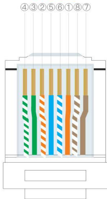
T568A
