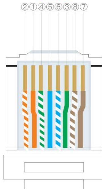
T568B
