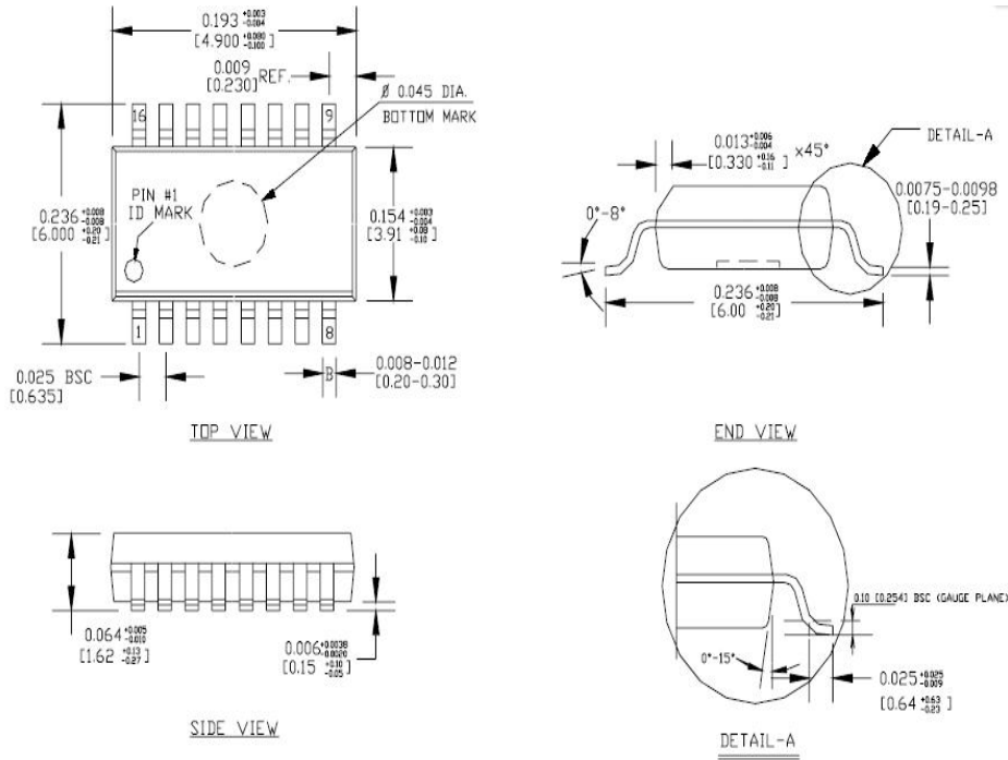
图 12 SSOP16 封装图
