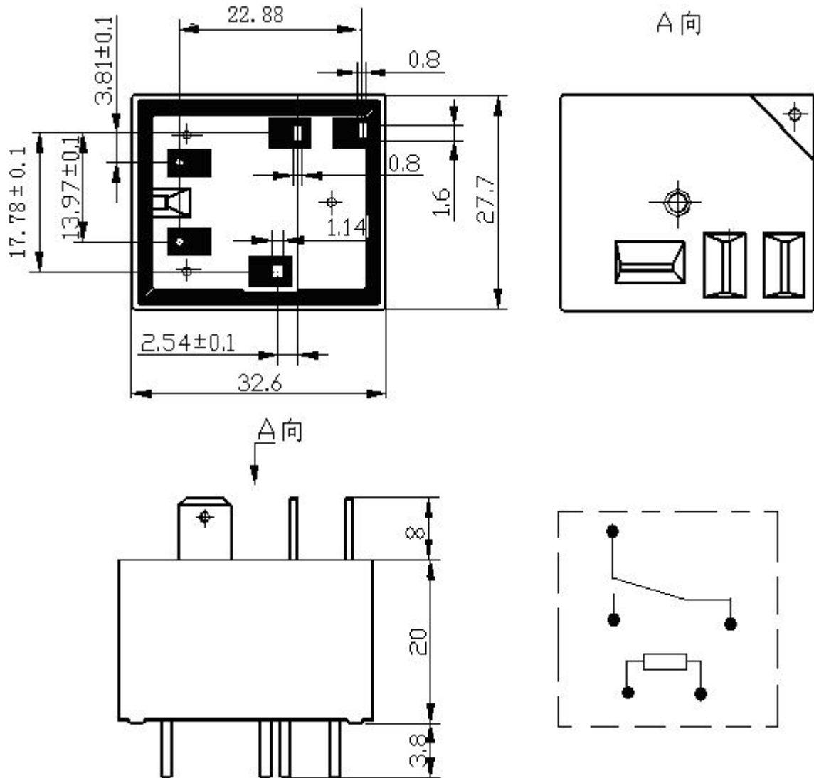
外形图
