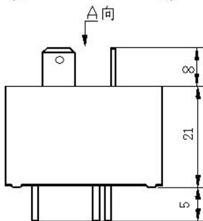
外形图
