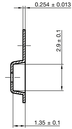
A-A Section
