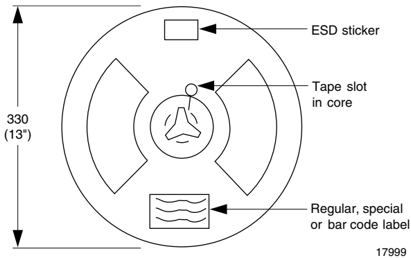
Fig. 22 - Reel Dimensions
