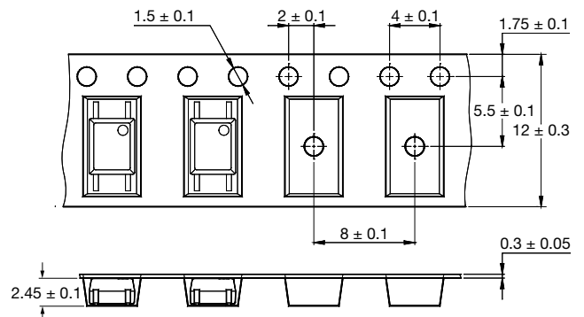
Fig. 17 - Tape Dimensions
