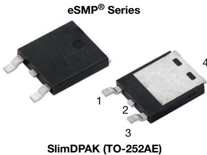
SlimDPAK (TO-252AE)
