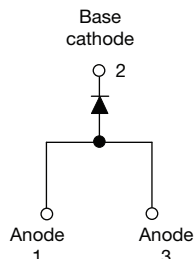
TO-247AC 3L
