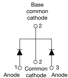
VS-40CTQ045-1-M3
