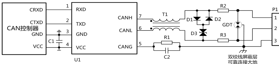
图 4. EMC 推荐电路
