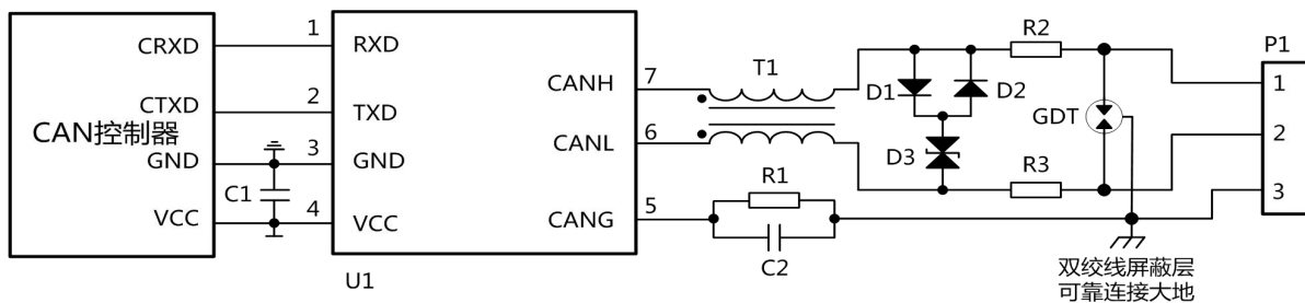
图 4. EMC 推荐电路
