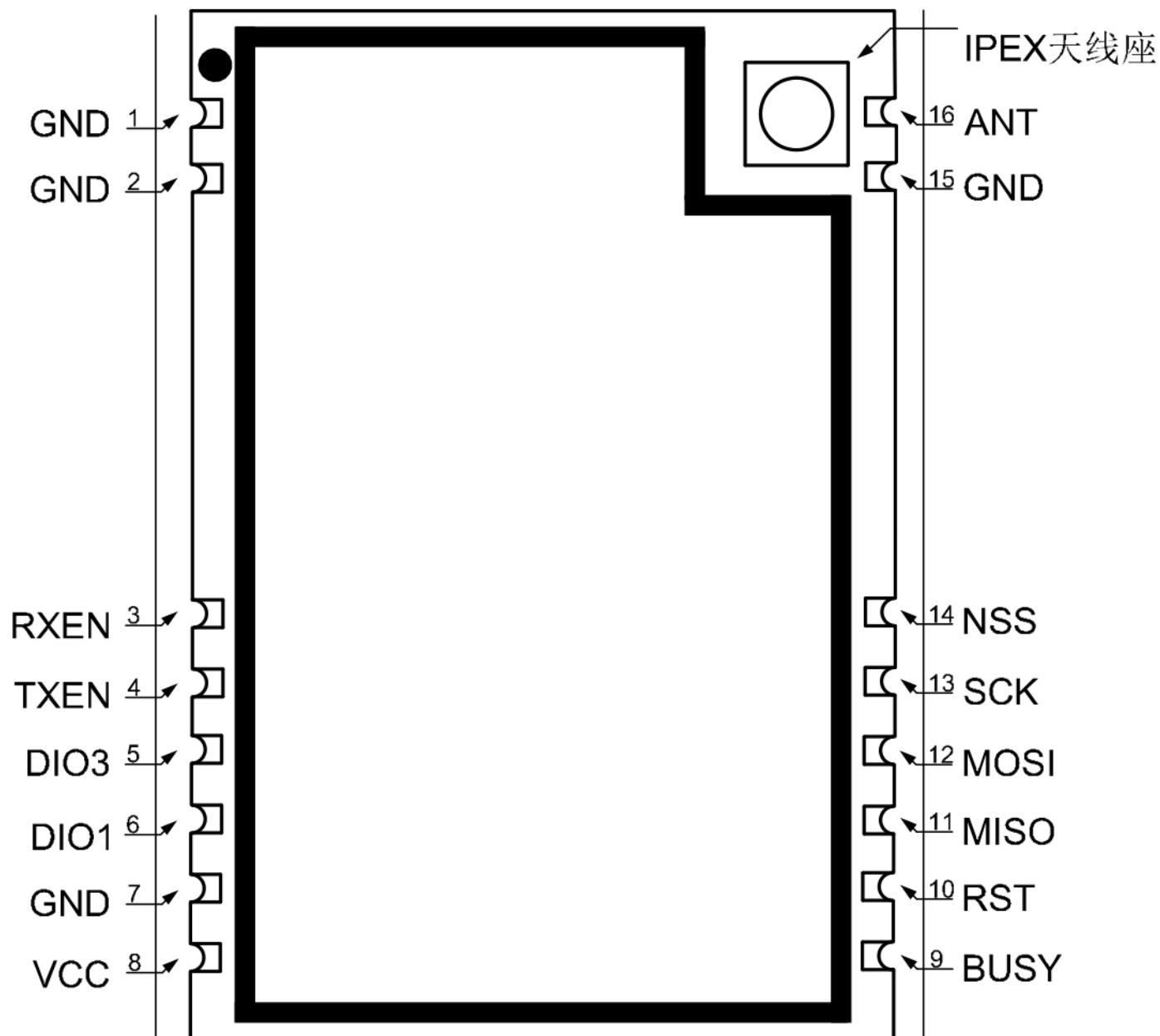
图 3-1 正面视图
