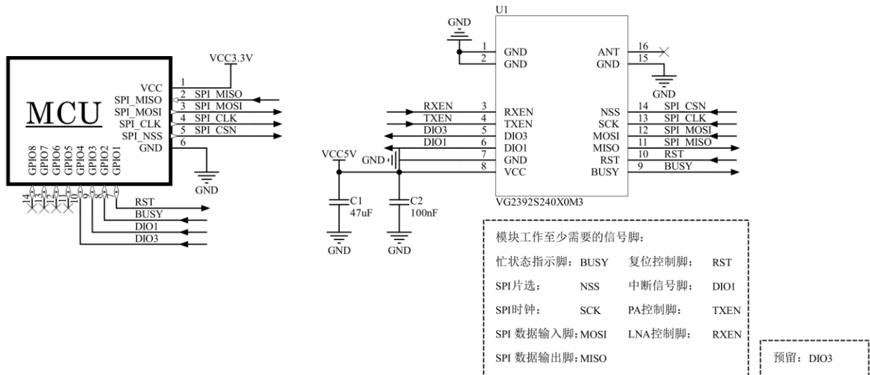
图 5-1、MCU 连接示意图
