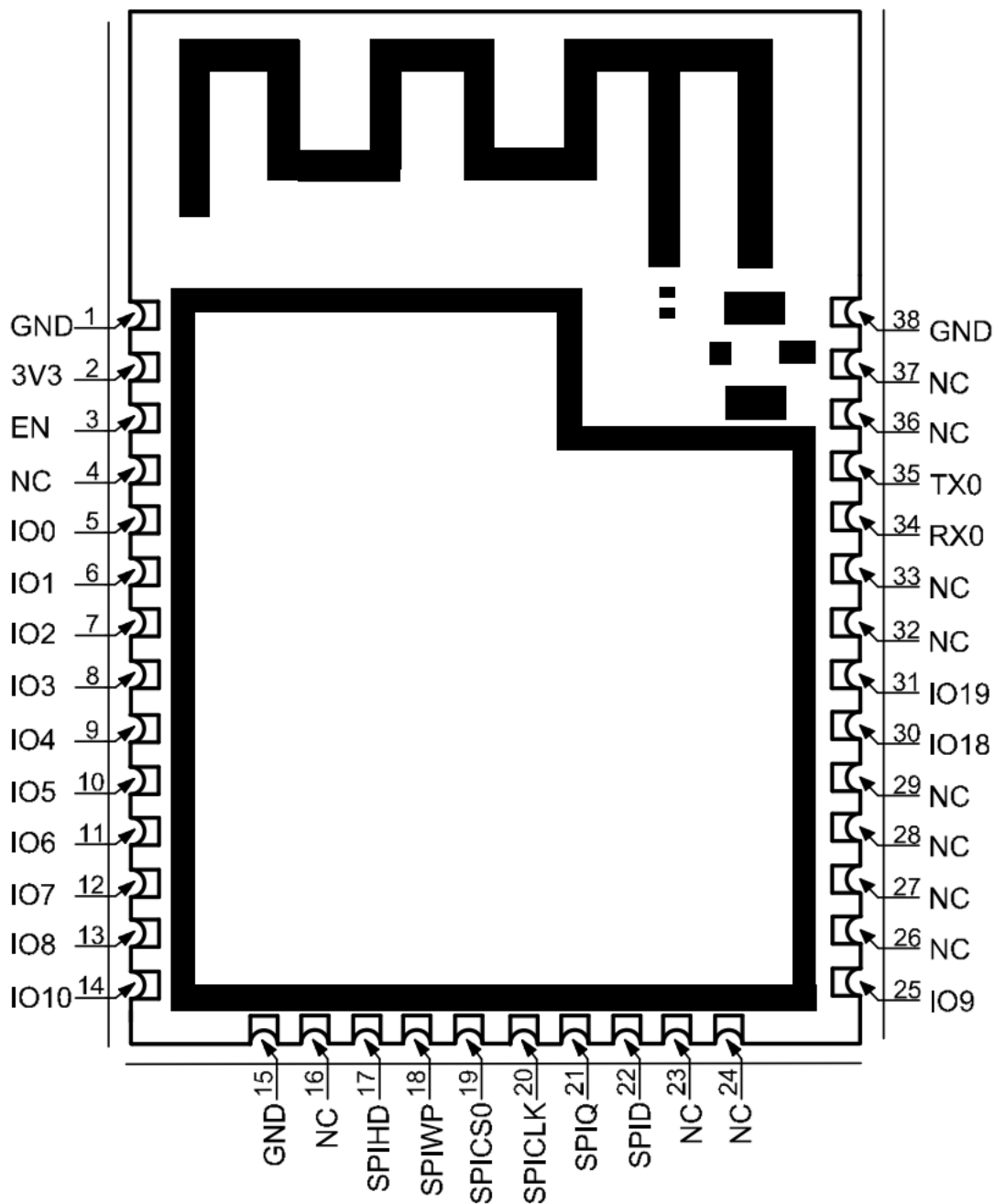
图 3-1 俯视图
