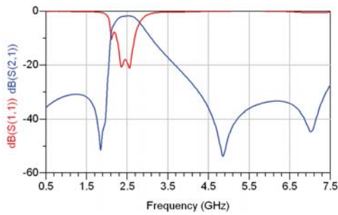
RFBPF2012080ADT
