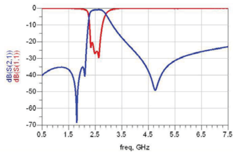
RFBPF2012080AGT
