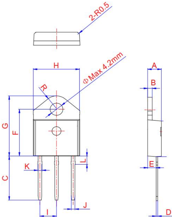
TO-3P Ins
