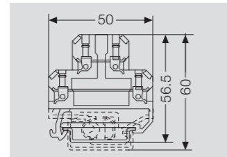
DK 5 U
