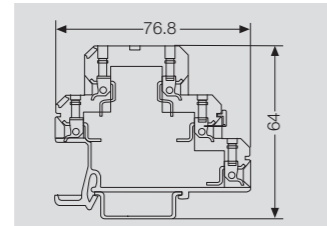
DK 6 U
