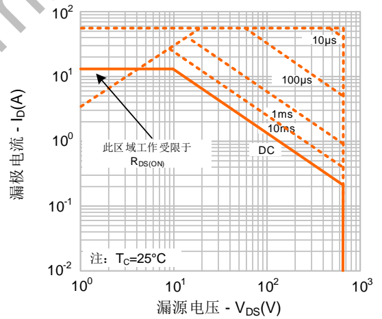
图9-2. 最大安全工作区域
