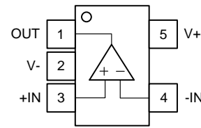
SOT-23-5L
