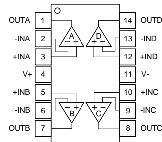
SOP-14L/TSSOP-14L
