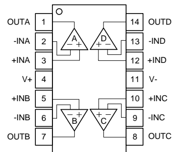
SOP-14L/TSSOP-14L
