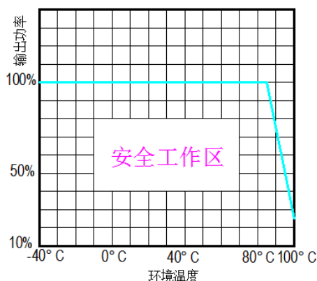
温度曲线图
