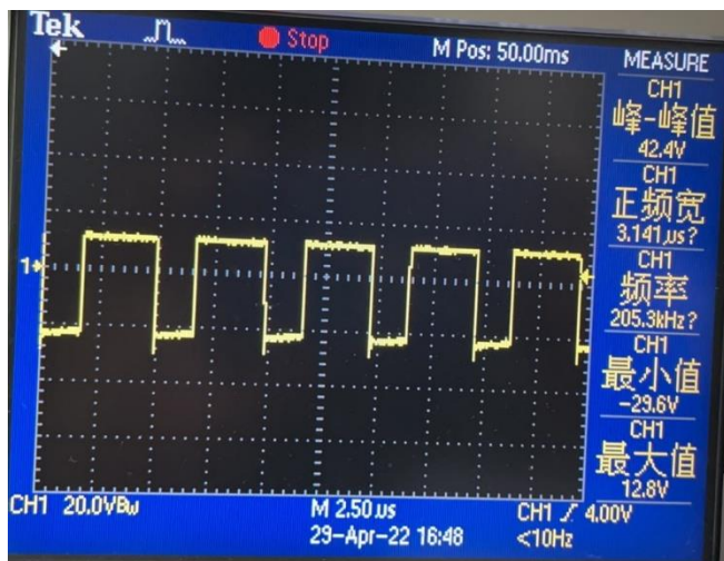
Rectifier diode
