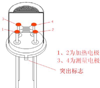
图 8： 管脚示意图
