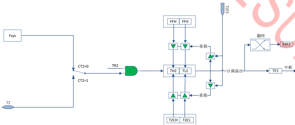
图 7.4.3-2 定时器 2 的重载模式 1
