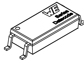
Scale - 4:1
