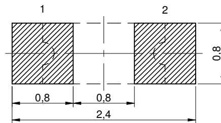
Scale - 20:1
