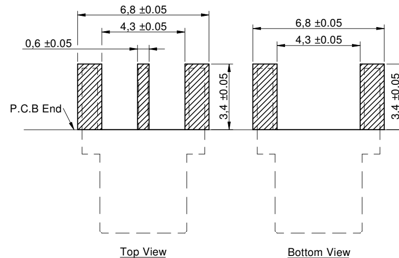
P.C.B Thickness: 1,6 mm
