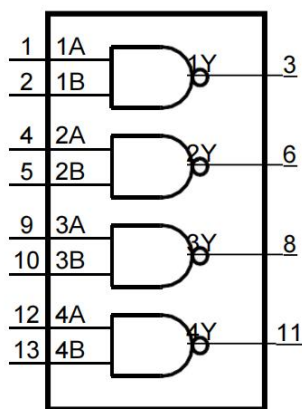
图 1 逻辑符号
