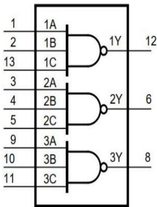
图1 逻辑符号
