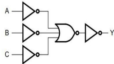
图3 逻辑框图
